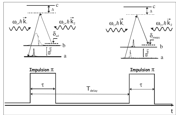
Fig. 3. – Protocole de mesure de vitesse. À chaque impulsion laser \pi est associée un schéma des niveaux atomiques et la distribution de vitesse associée dans chaque niveau d'énergie après la transition Raman.
