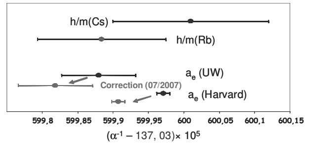
Fig. 1. – Les principales déterminations de la constante de structure fine \alpha retenues par le CODATA 2006 pour l'ajustement de la valeur recommandée. Les valeurs fléchées représentent les valeurs corrigées suite à une révision des calculs de l'électrodynamique quantique.
